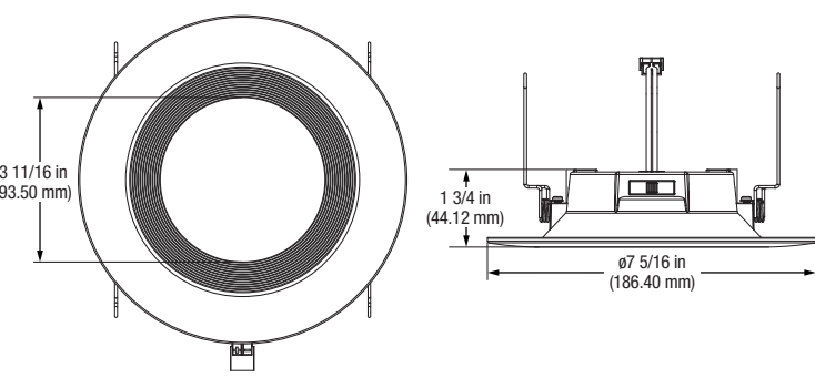
6" BAFFLE
