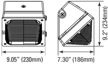
28W 5.51-lbs
