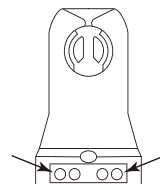
Portalámparas sin resistencia de derivación.
