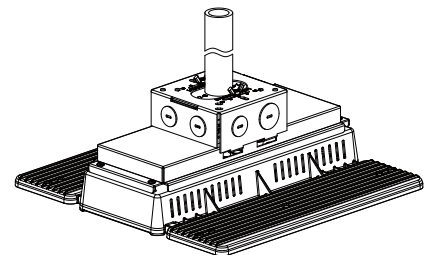
Pendant Mounting
