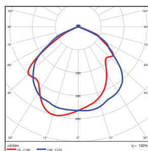
LED9PL- Horizontal
