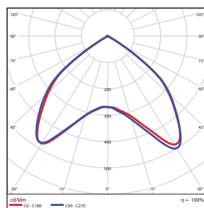
LED9PL- Vertical
