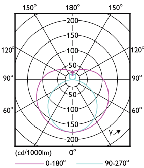
LEDtube COR NAM4 25W G5 3300lm-LDD
