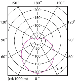
Light Distribution Diagram - 10A19/CNG/830/FR/P/E26/ND 4/1CT
