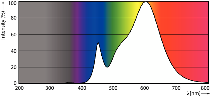
Spectral Power Distribution Colour - 10A19/CNG/830/FR/P/E26/ND 4/1CT
