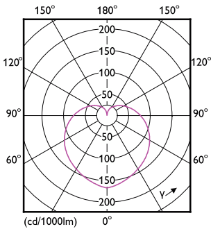
Light Distribution Diagram - 5A19/CNG/850/FR/P/E26/D 12/1CT
