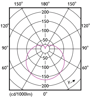
Light Distribution Diagram - 5A19/CNG/840/FR/P/E26/D 12/1CT
