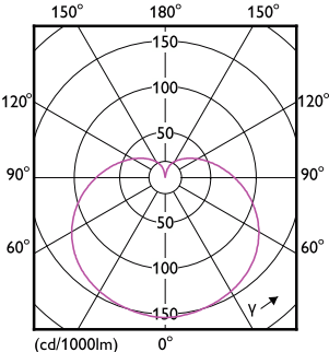
Light Distribution Diagram - 5A19/CNG/827/FR/P/E26/D 12/1CT
