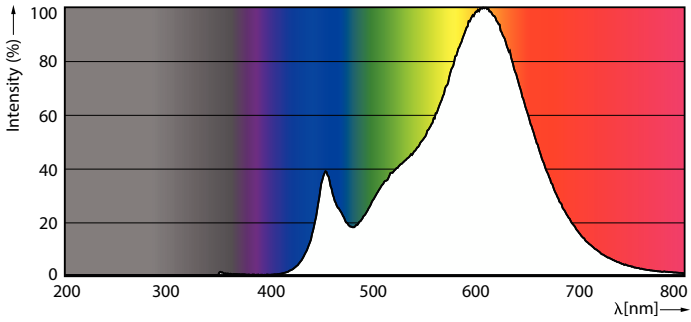
Spectral Power Distribution Colour - 5A19/CNG/827/FR/P/E26/D 12/1CT
