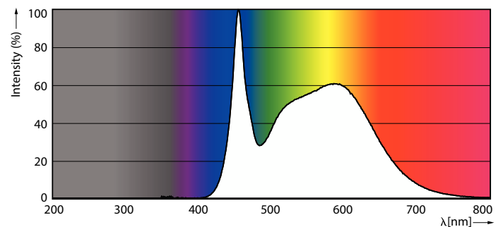
Spectral Power Distribution Colour - 14A19/CNG/850/FR/P/E26/D 12/1CT
