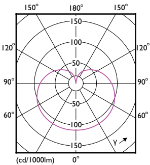
Light Distribution Diagram - 8.8A19/CNG/840/FR/P/E26/D 12/1CT
