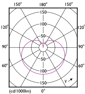
Light Distribution Diagram - 8.8A19/CNG/830/FR/P/E26/D 12/1CT
