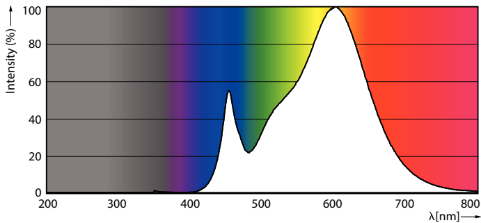
Spectral Power Distribution Colour - 9A19/CNG/830/FR/P/E26/ND 4/1CT
