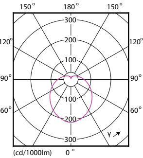
Light Distribution Diagram - 9A19/CNG/830/FR/P/E26/ND 4/1CT
