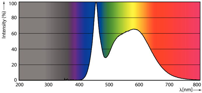
Spectral Power Distribution Colour - 10A19/CNG/850/FR/P/E26/ND 4/1CT
