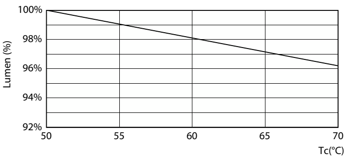
LEDtube COR 8ft 33W 50K LumenVsTc-LMP
