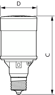
80CC/LED/840/LS EX39 G2 BB 3/1
