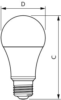
A19 120V 12.2-75W 1100lm 4000K E26 D
