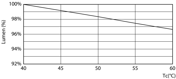
LEDtube_70K_LumenVsTc-LMP
