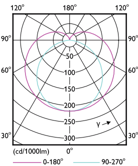
LEDtube_G13_1-LDD
