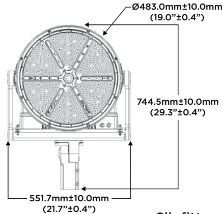
Slipfitter
