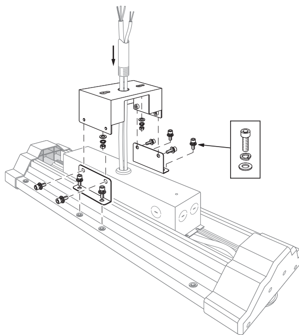
PENDANT MOUNTING*
