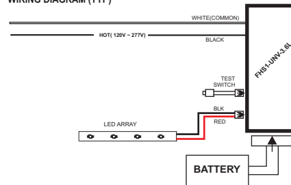
WIRING DIAGRAM (TYP)
