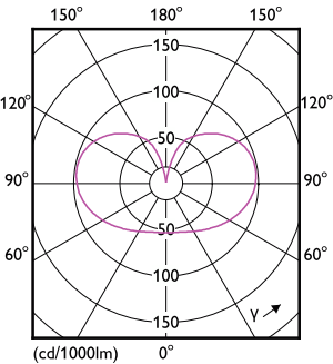
Light Distribution Diagram - 8A19/PER/UD/FR/G/E26/WGD 4/2PFT20
