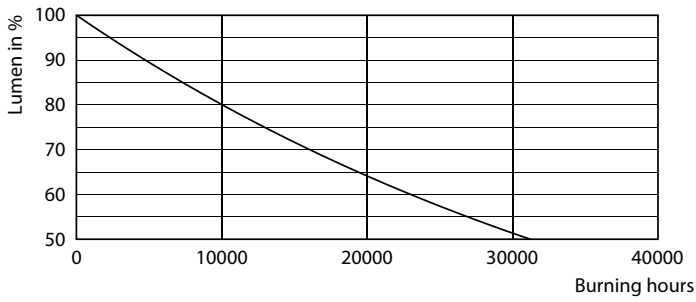
Lumen Maintenance Diagram - 4A19/PER/PURPLE/G/E26/ND 4/1PF
