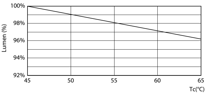
LEDtube_70K_1_LumenVsTc-LMP
